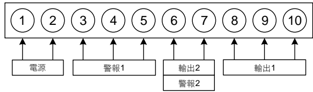
下排端子
