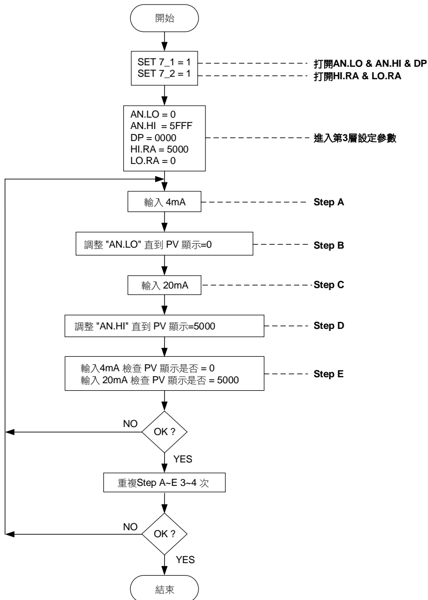
Input 信號 (4mA~20mA) 校正流程圖
