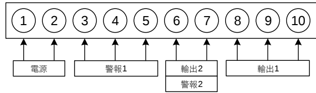
下排端子
